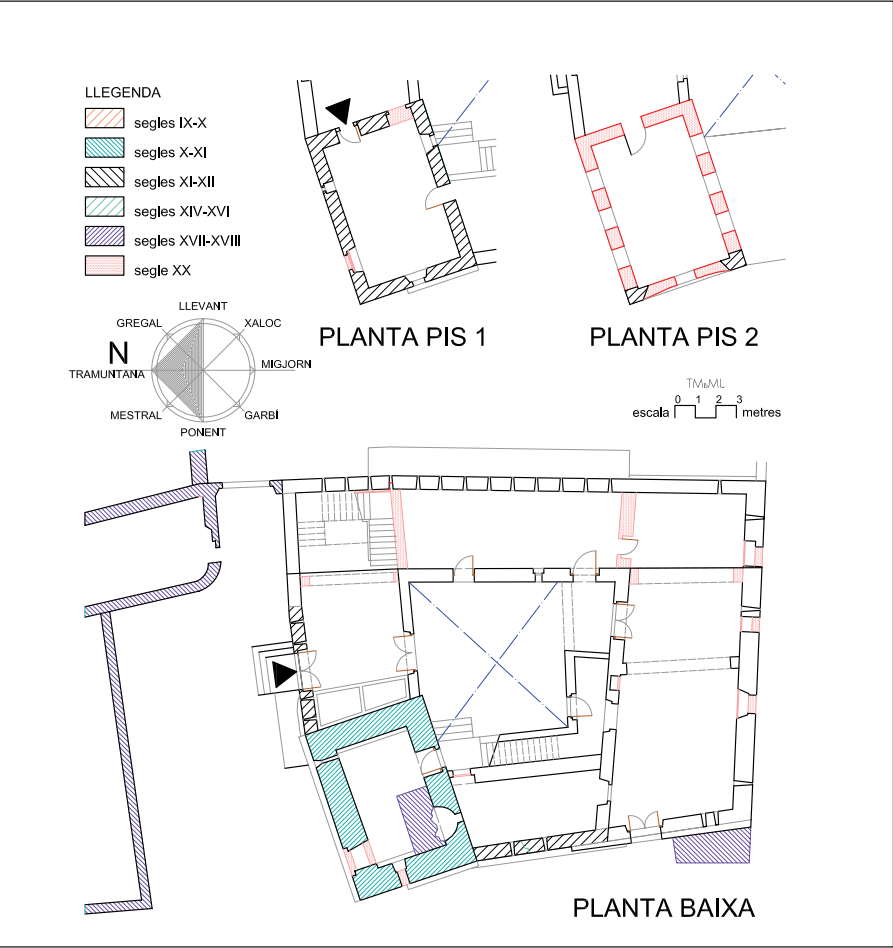
CASTELL DE PLEGAMANS. Planta baixa del castell i planta primera i segona de la torre.
