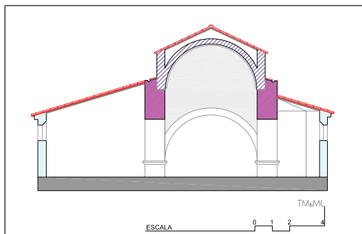
SANTA MARIA DE PALAU-SOLITÀ. Secció transversal de l'església.
