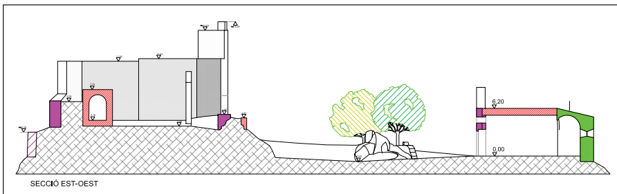
CASTELL DE MONTBUI. Secció del castell i de la capella de Sant Mateu.
