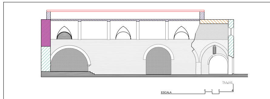
SANTA MARIA DE PALAU-SOLITÀ. Secció longitudinal on podem veure les diferents reformes que ha sofert al llarg dels anys.
