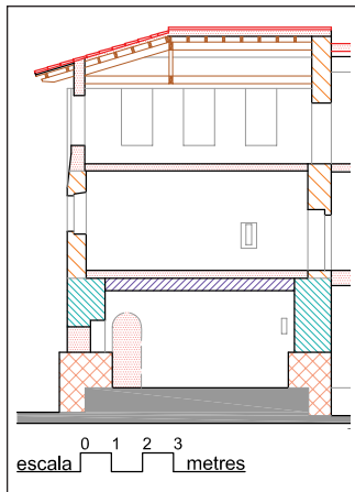
CASTELL DE PLEGAMANS. Secció de la torre mirant a tramuntana.
