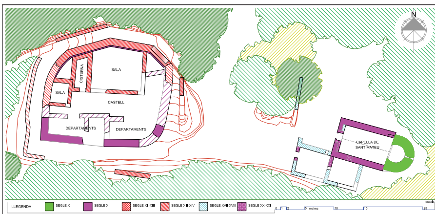
CASTELL DE MONTBUI. Planta del castell i de la capella de Sant Mateu.
